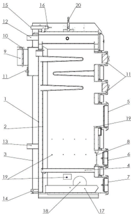
Рис. 1. Схема конструкції котлів ЕКО – KWRW 60 і 70
