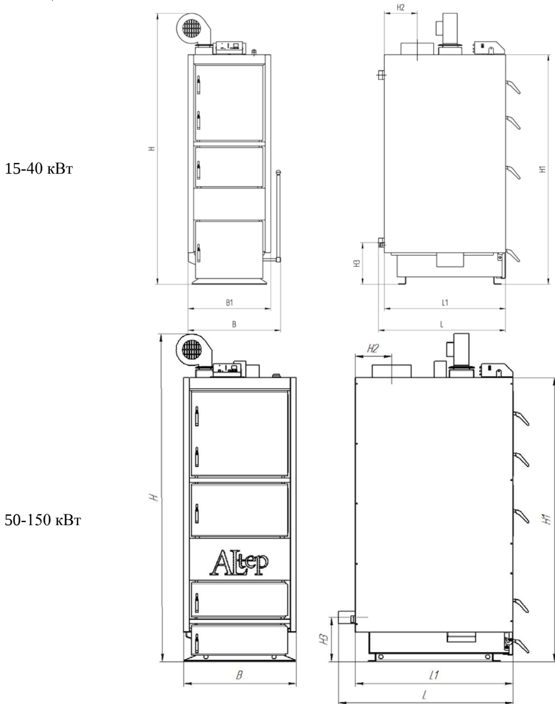
Рисунок 1 – Габаритне креслення котла типу КТ-2-Н
