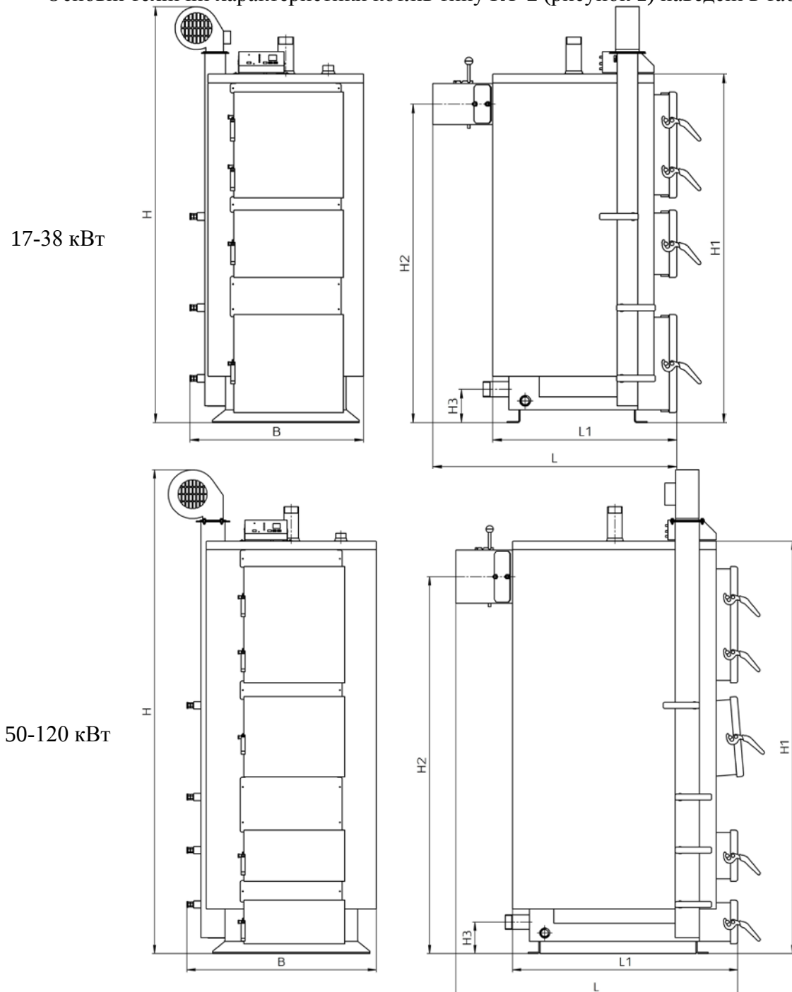
Рисунок 1 – Габаритне креслення котла типу КТ-2
