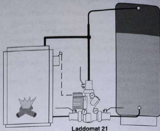
Laddomat 21
